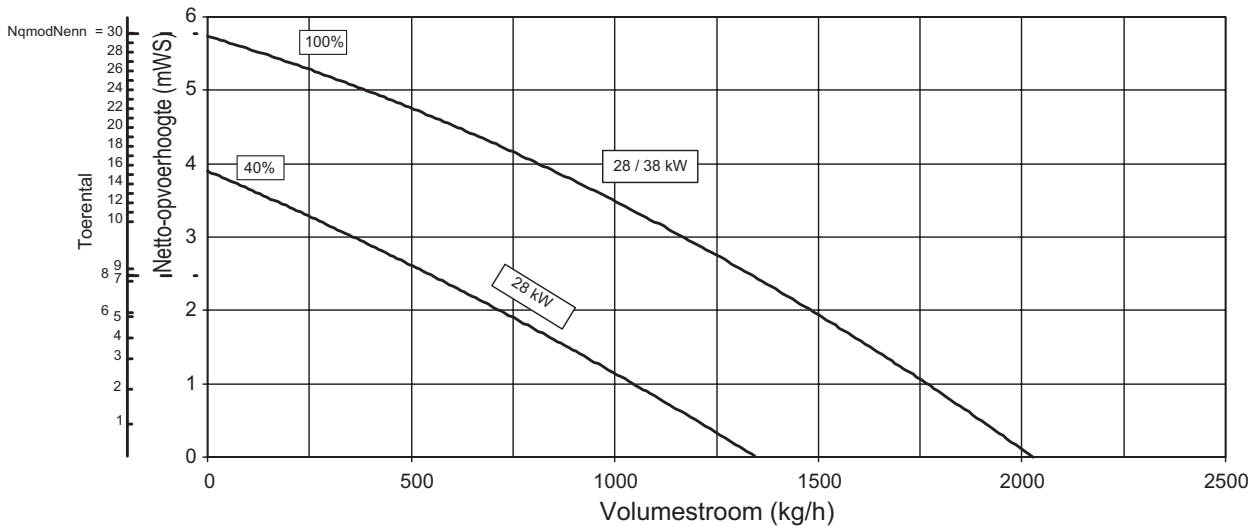
Abb. 10 Netto-opvoerhoogte
