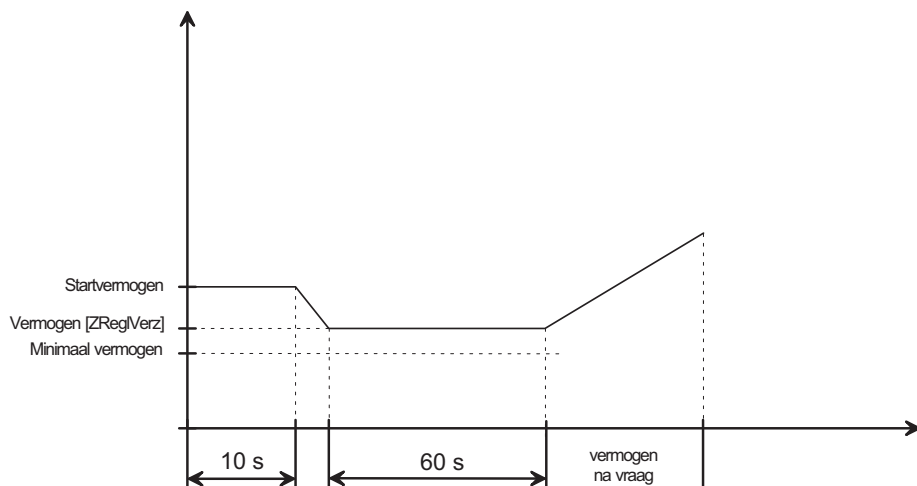
Schets 10 Werkingsverloop na het starten van de brander
