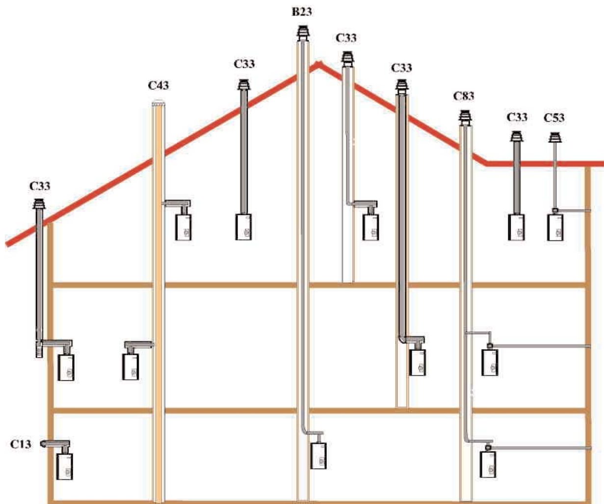
Schets. 6 Opstel mogelijkheden met de BAXI-MG (accessoires)
