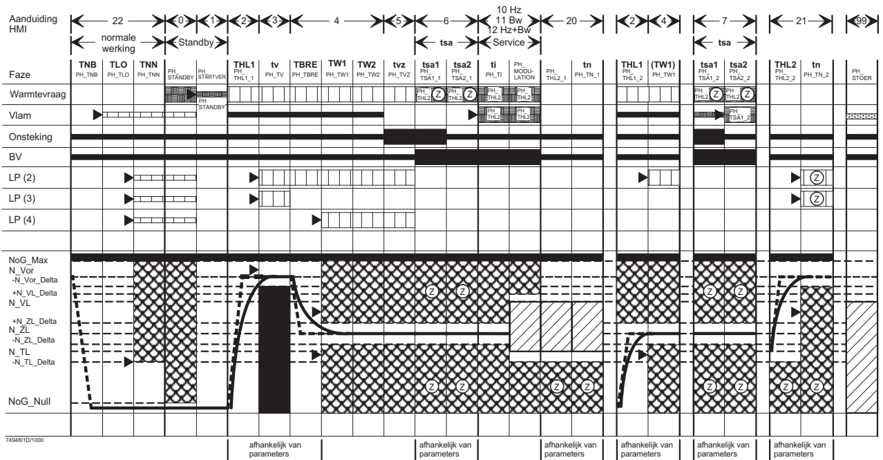
Schets 14 Verloop van de sturings- en regelcentrale BMU (type LMU64.00x/A100)
