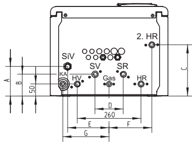
Schets. 1 Afmetingen en aansluitingen
